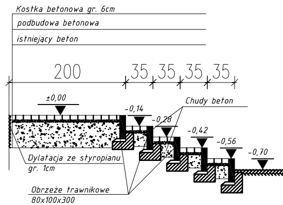
PRZEKRÓJ B-B
